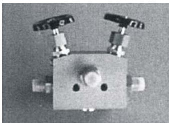
Blok zaworowy do stacji ręcznego przełączania
