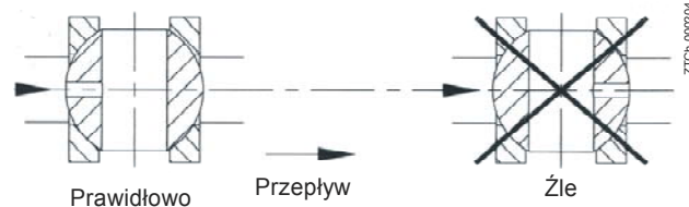
Rys. 3. Montaż zaworów
