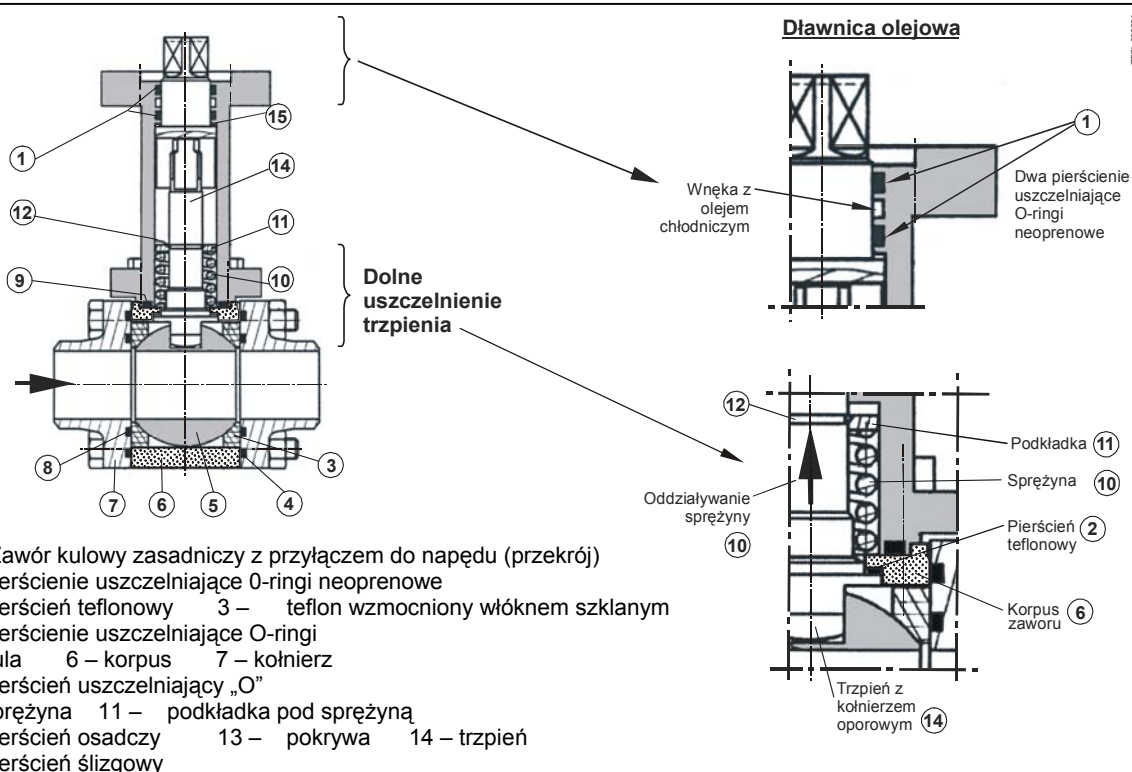
Rys.1. Zawór XAD
