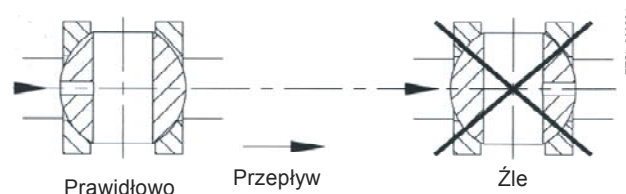
Rys. 3. Montaż zaworów
