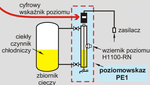
Wyświetlacz poziomowskazu
