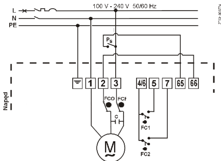
Rys.11. Przykładowy schemat połączeń elektrycznych zaworów z zasilaczem awaryjnym. W wypadku zaniku napięcia zasilania następuje zamknięcie zaworu. Opcyjnie dostępne napędy o działaniu odwrotnym.
