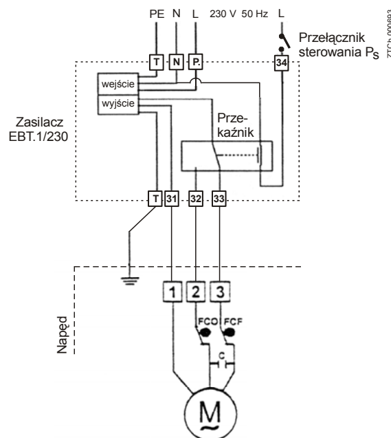
Rys. 12. Przykład połączenia zaworu i zasilacza awaryjnego. Pozostałe połączenia zgodnie ze schematem na Rys. 9 i Rys.10. Grzałka musi być podłączona zawsze, na stałe.
