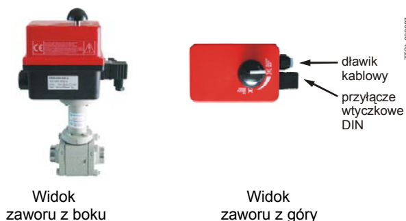
Rys. 6. Wejścia elektryczne napędów
