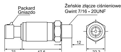
Packard żeńskie Wymiary w mm
