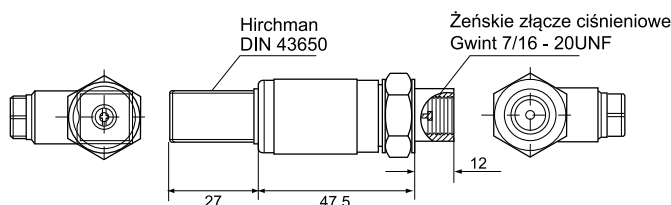
Hirschman żeńskie Wymiary w mm
