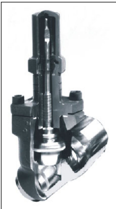
Zawór regulacyjny półhermetyczny RCDS (przekrój). Trzpień zakryty kapturkiem uszczelniającym
